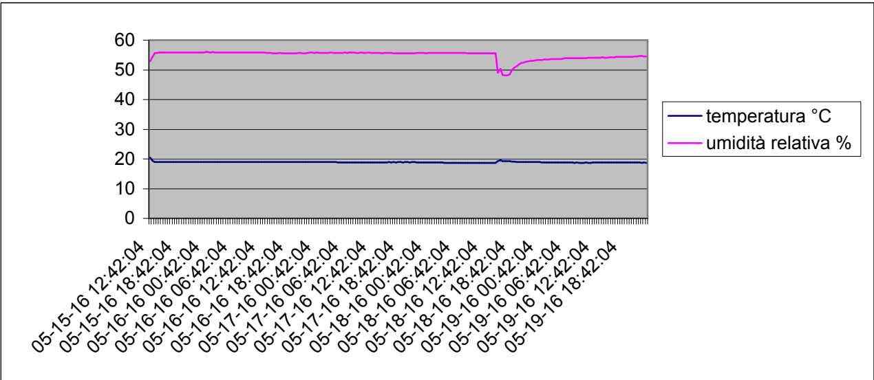
Grafico della temperature e dell'umidità relativa interna dal 15-05-2016 al 19-05-2016
