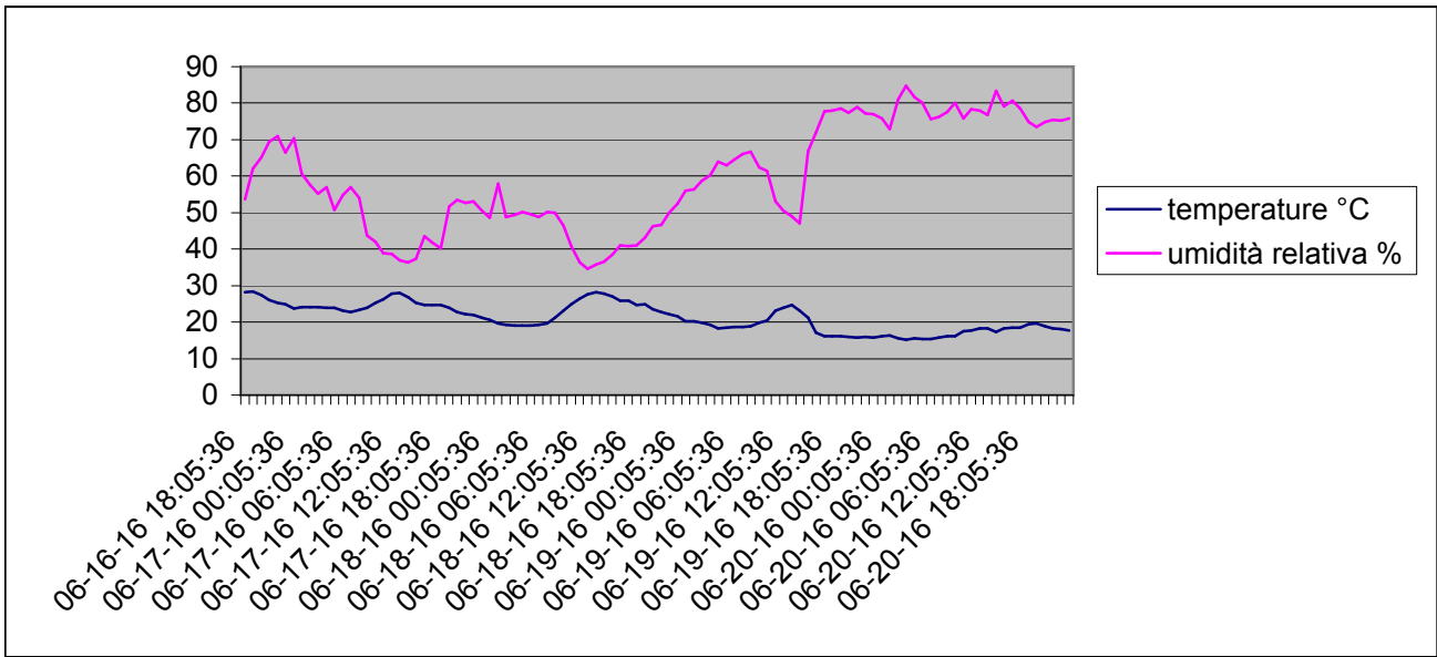
Grafico della temperature e dell'umidità relativa esterna dal 21-06-2016 al 26-06-2016
