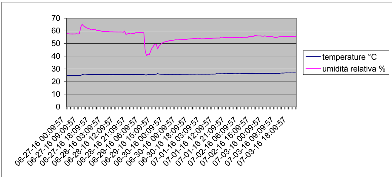
Grafico della temperature e dell'umidità relativa interna dal 27-06-2016 al 3-07-2016
