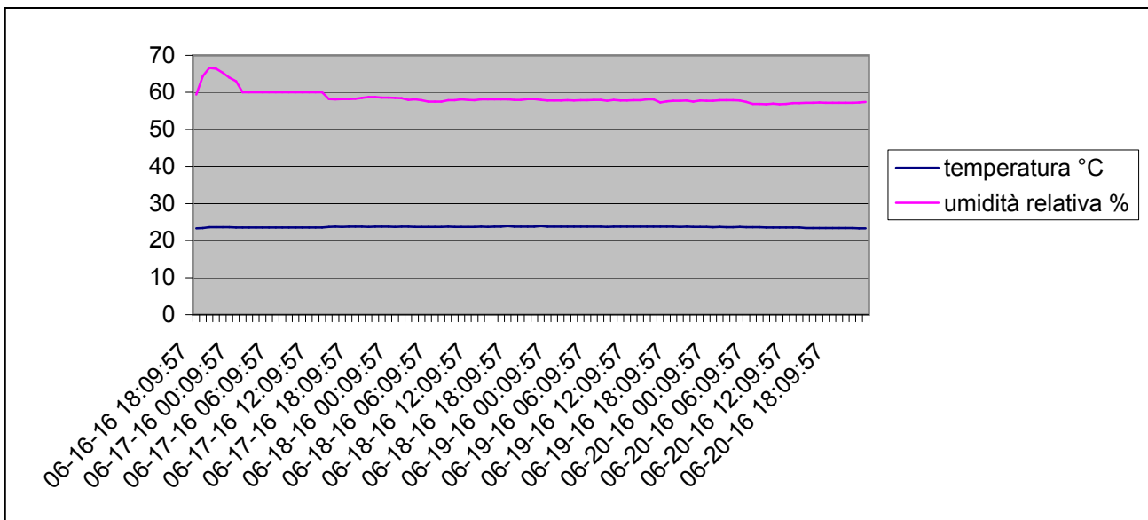
Grafico della temperature e dell'umidità relativa interna dal 21-06-2016 al 26-06-2016
