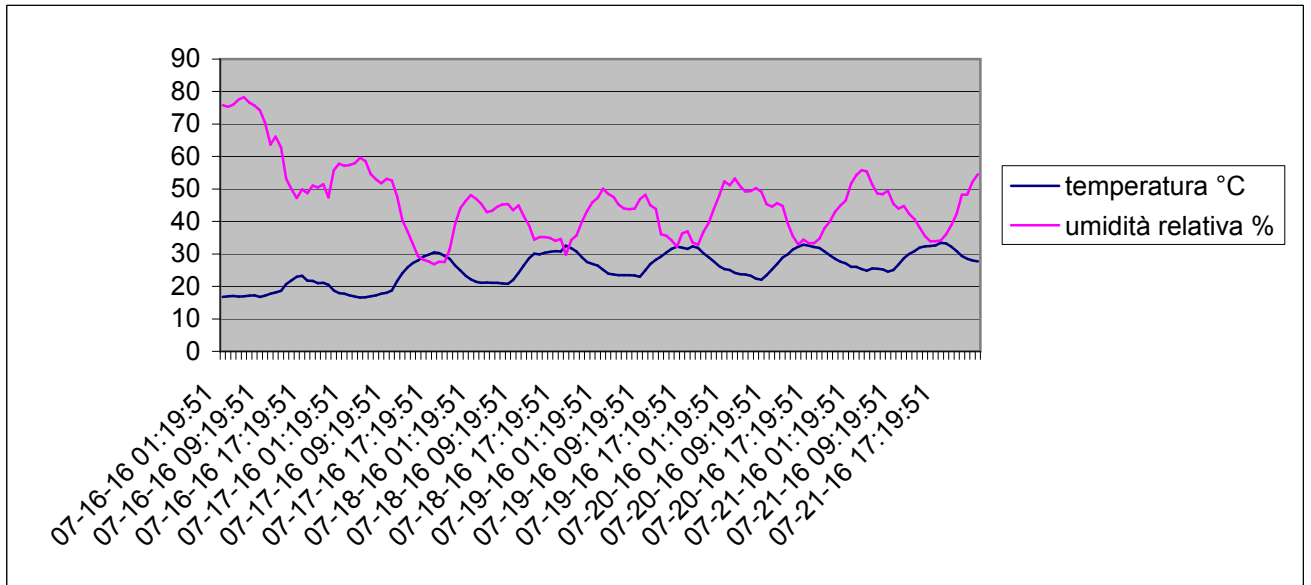
Grafico della temperature e dell'umidità relativa esterna dal 16-07-2016 al 21-07-2016
