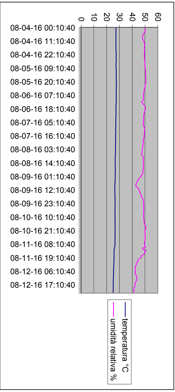
Grafico della temperature e dell'umidità relativa interna dal 4-08-2016 al 12-08-2016
