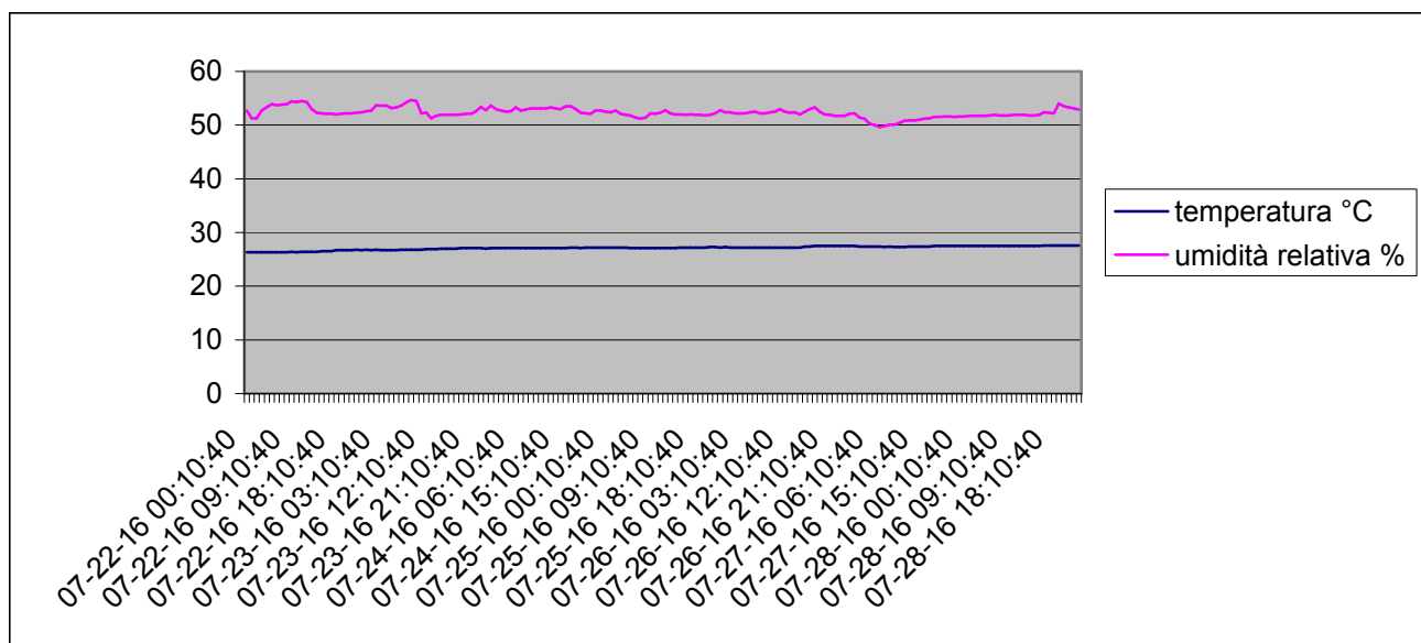
Grafico della temperature e dell'umidità relativa interna dal 22-07-2016 al 28-07-2016
