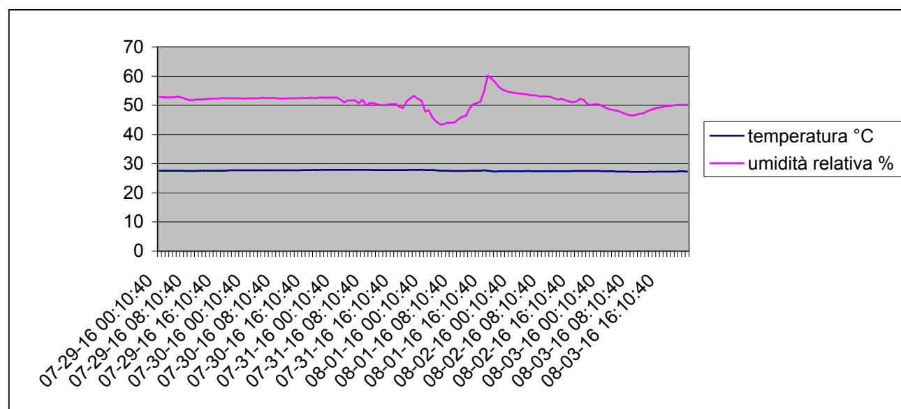
Grafico della temperature e dell'umidità relativa interna dal 29-07-2016 al 3-08-2016
