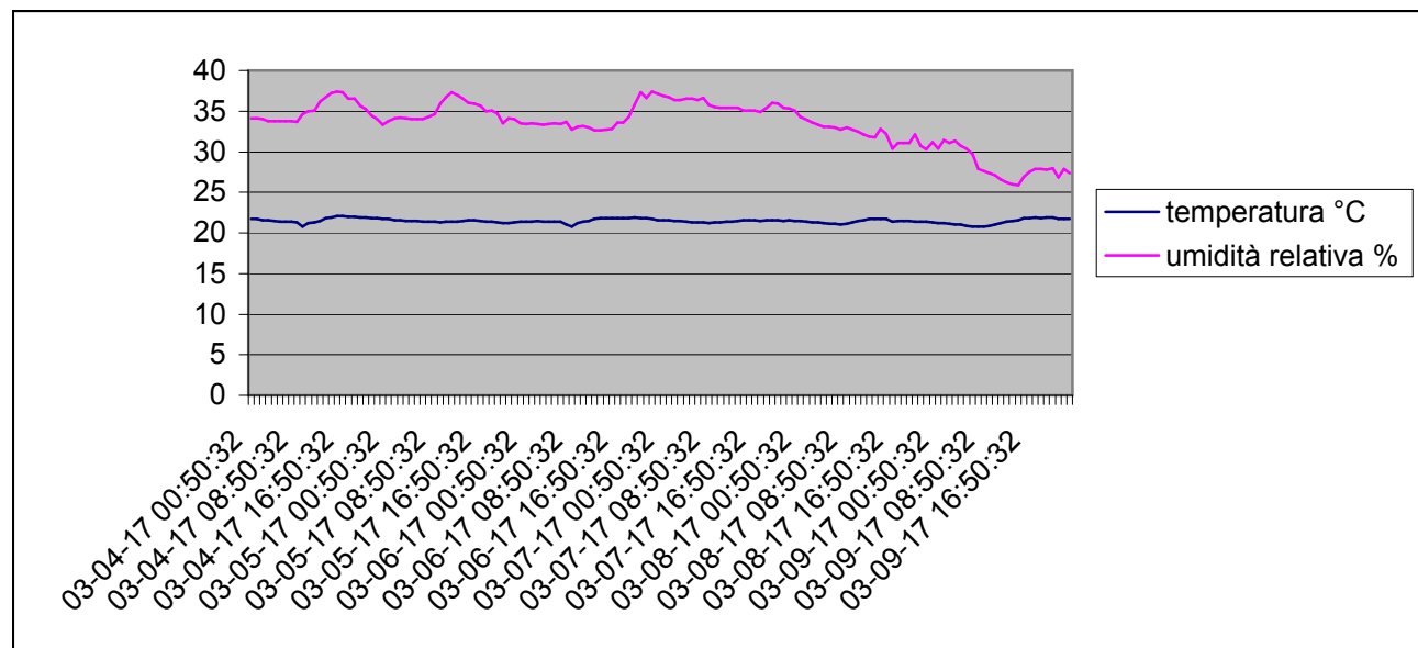
Grafico della temperature e dell'umidità relativa interna dal 4-3-2017 al 9-3-2017
