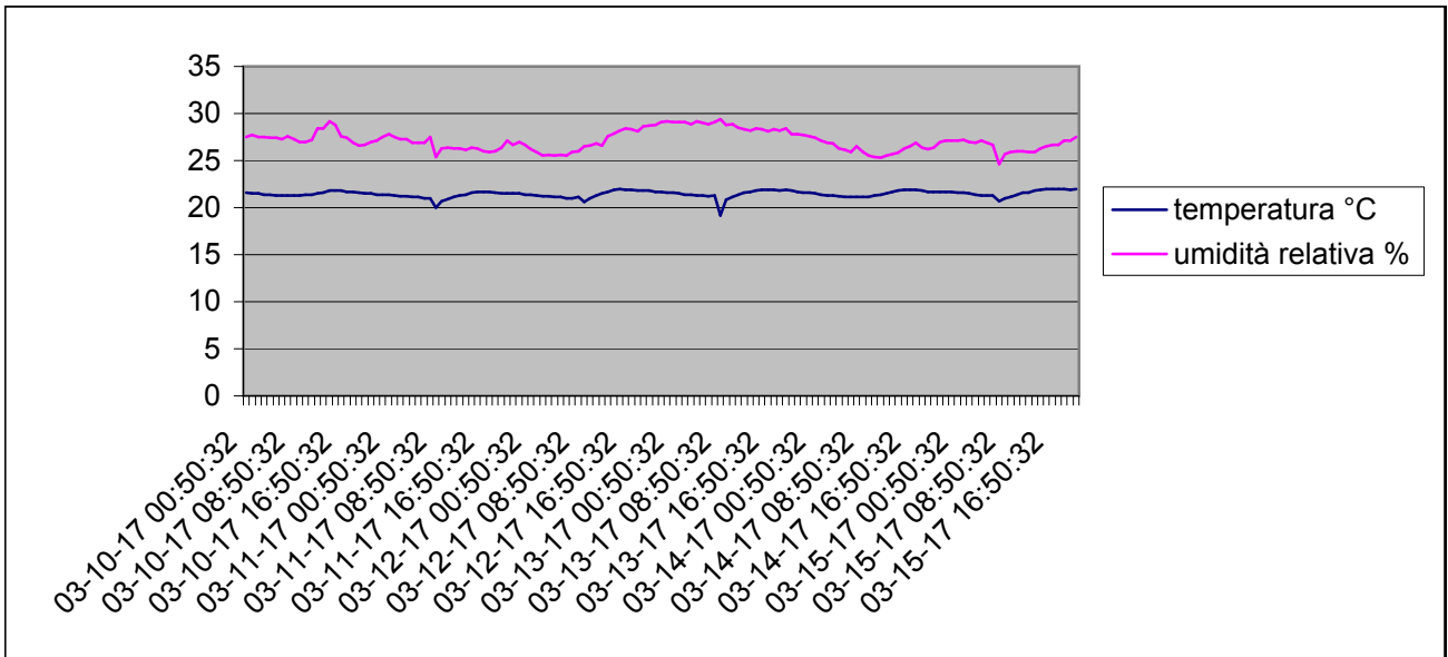
Grafico della temperature e dell'umidità relativa interna dal 10-3-2017 al 15-3-2017
