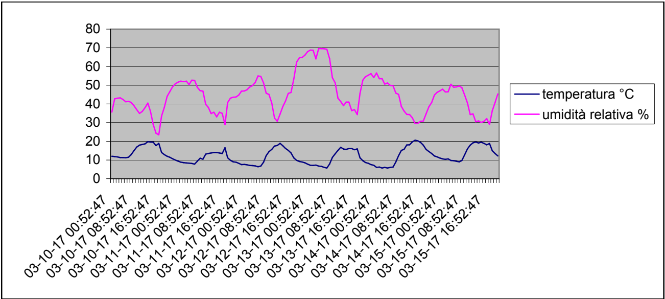
Grafico della temperature e dell'umidità relativa esterna dal 10-3-2017 al 15-3-2017
