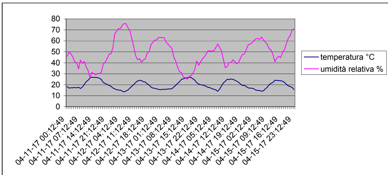
Grafico della temperature e dell'umidità relativa esterna dal 11-4-2017 al 15-4-2017
