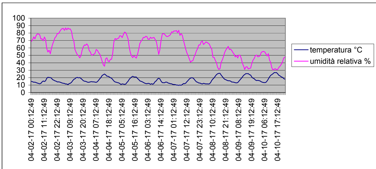
Grafico della temperature e dell'umidità relativa esterna dal 2-4-2017 al 10-4-2017
