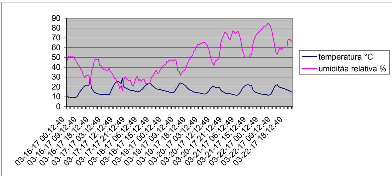
Grafico della temperature e dell'umidità relativa esterna dal 16-3-2017 al 22-3-2017
