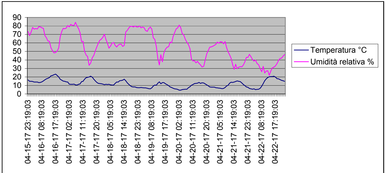
Grafico della temperature e dell'umidità relativa esterna dal 16-4-2017 al 22-4-2017
