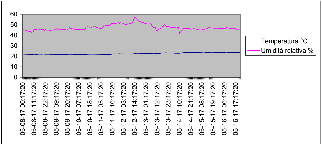
Grafico della temperature e dell'umidità relativa interna dal 8-5-2017 al 16-5-2017
