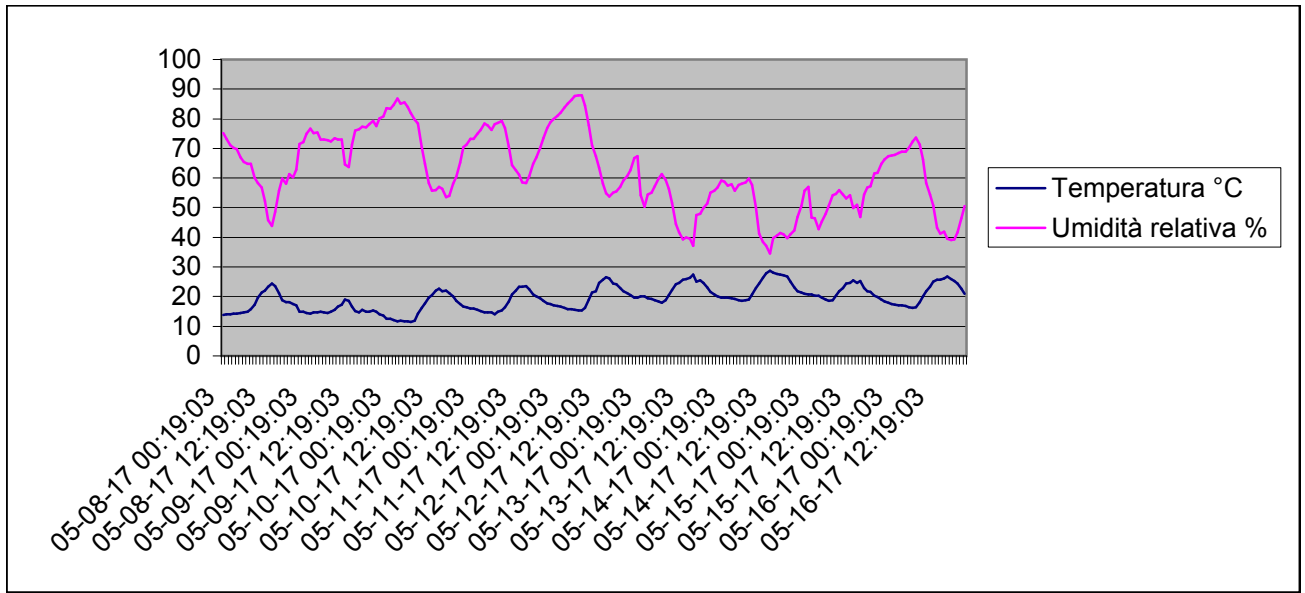
Grafico della temperature e dell'umidità relativa esterna dal 8-5-2017 al 16-5-2017
