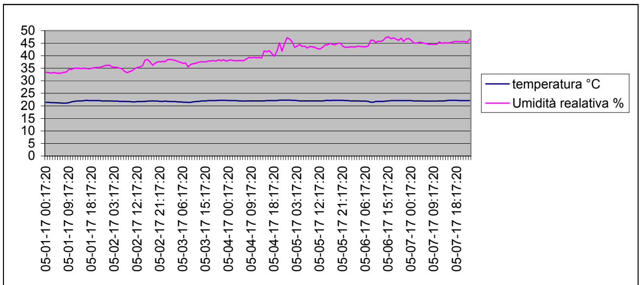
Grafico della temperature e dell'umidità relativa interna dal 1-5-2017 al 7-5-2017
