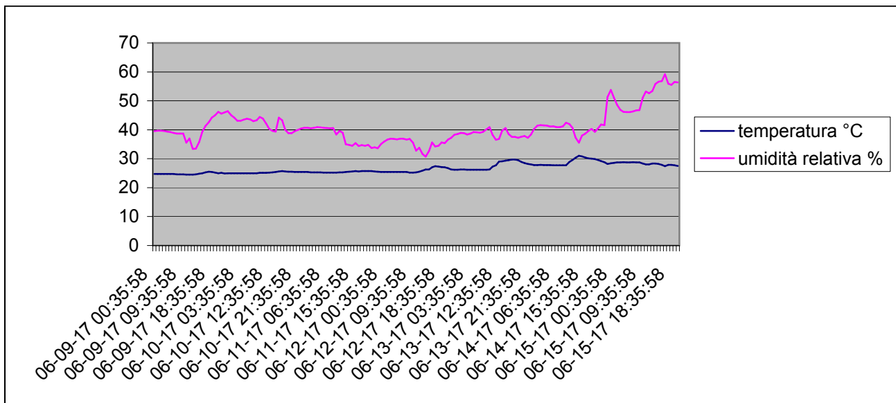
Grafico della temperature e dell'umidità relativa interna dal 9-6-2017 al 15-6-2017
