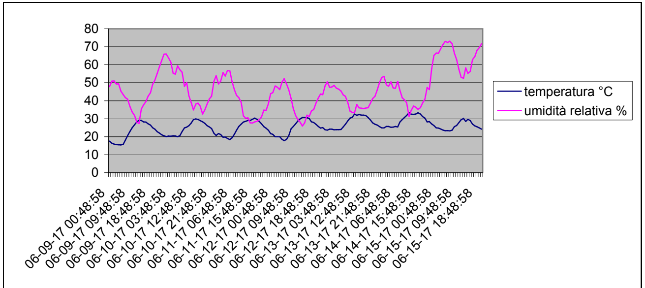
Grafico della temperature e dell'umidità relativa esterna dal 09-6-2017 al 15-6-2017
