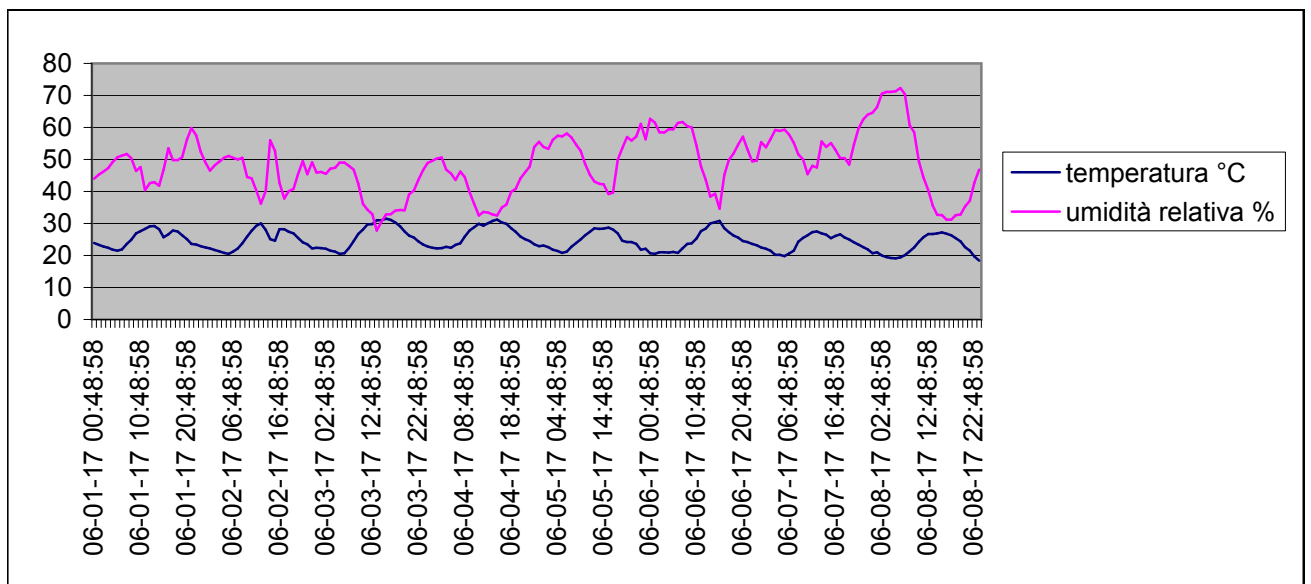
Grafico della temperature e dell'umidità relativa esterna dal 01-6-2017 al 8-6-2017
