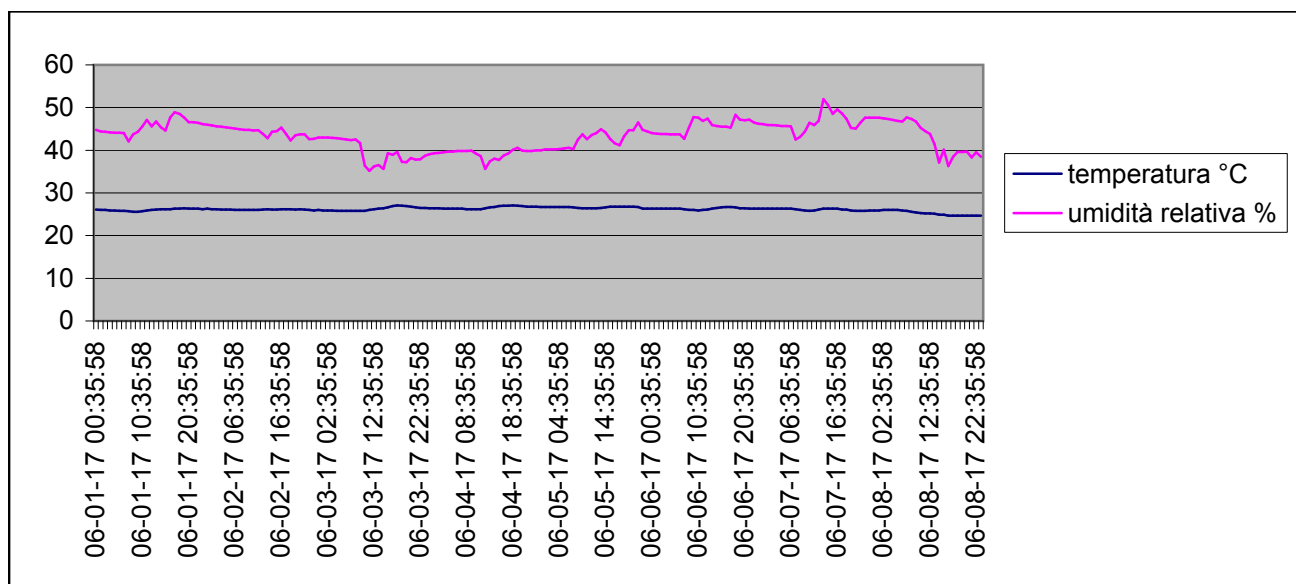
Grafico della temperature e dell'umidità relativa interna dal 1-6-2017 al 8-6-2017
