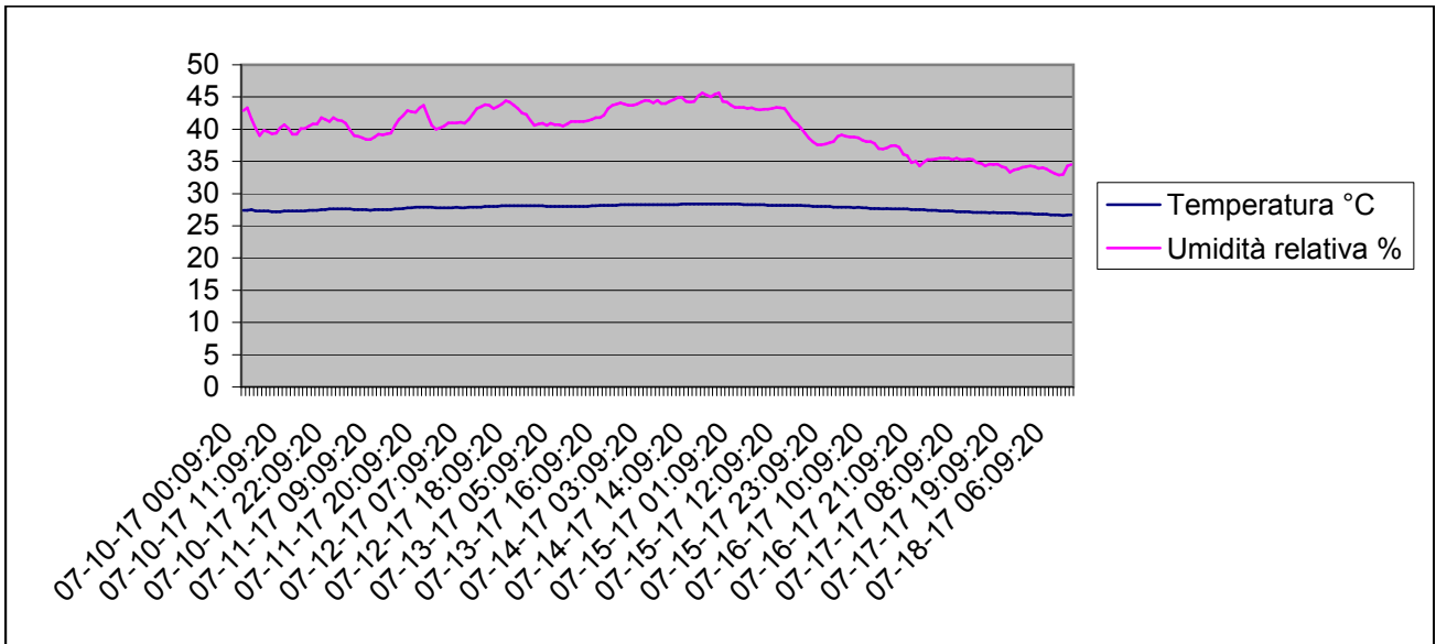
Grafico della temperature e dell'umidità relativa interna dal 10-7-2017 al 18-7-2017
