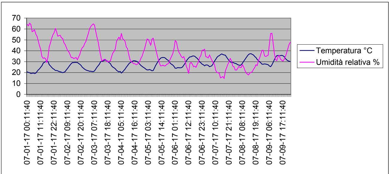
Grafico della temperature e dell'umidità relativa esterna dal 1-7-2017 al 9-7-2017
