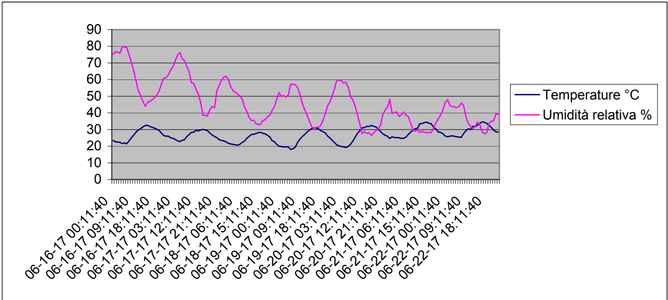
Grafico della temperature e dell'umidità relativa esterna dal 23-6-2017 al 30-6-2017
