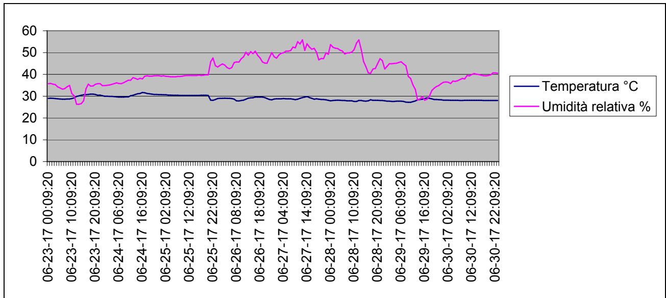
Grafico della temperature e dell'umidità relativa interna dal 23-6-2017 al 30-6-2017
