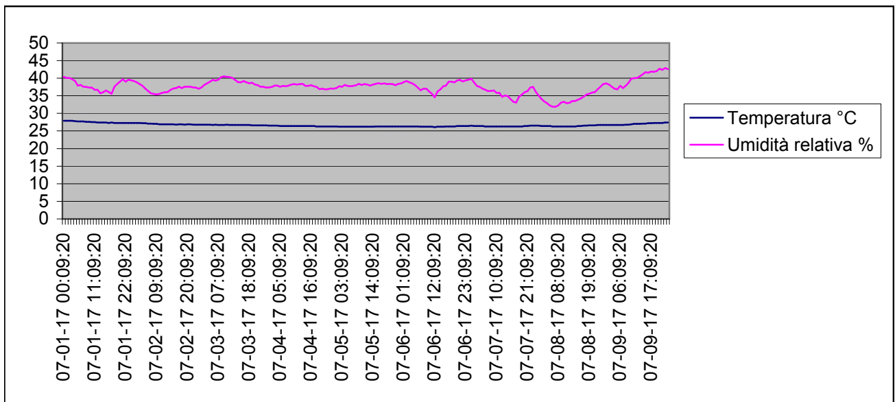
Grafico della temperature e dell'umidità relativa interna dal 1-7-2017 al 9-7-2017
