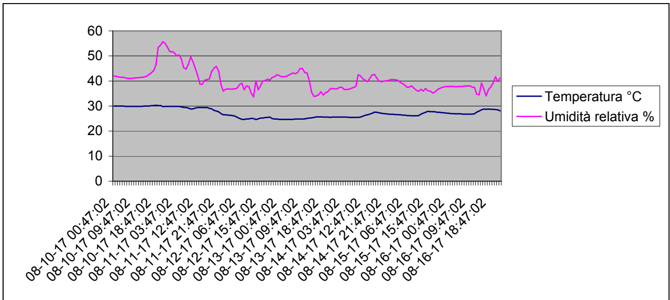
Grafico della temperature e dell'umidità relativa interna dal 10-8-2017 al 16-8-2017
