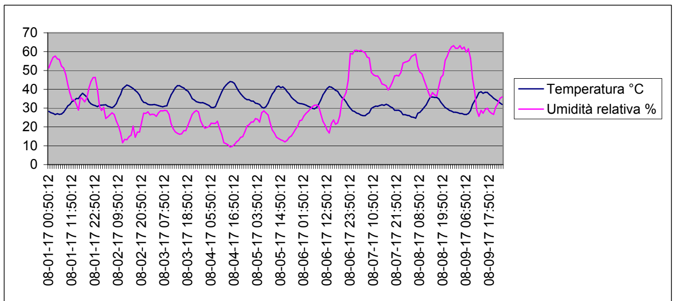
Grafico della temperature e dell'umidità relativa esterna dal 1-8-2017 al 9-8-2017
