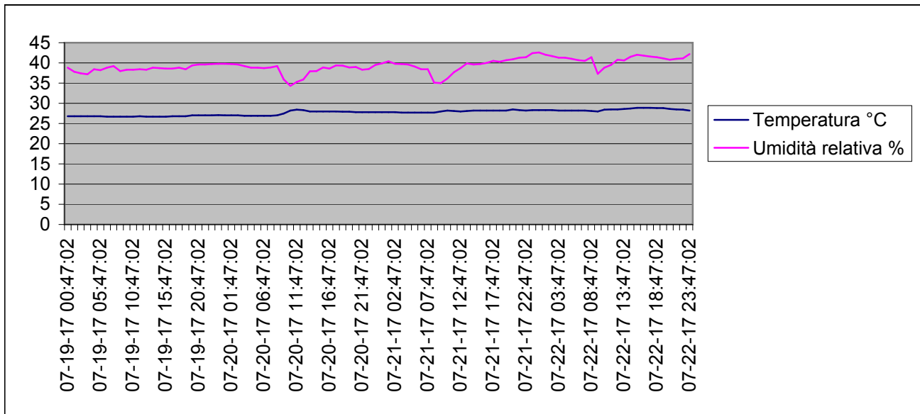
Grafico della temperature e dell'umidità relativa interna dal 18-7-2017 al 22-7-2017
