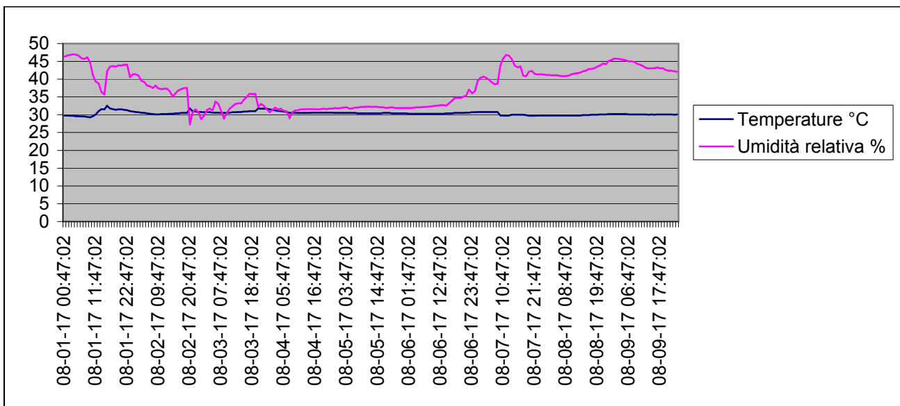
Grafico della temperature e dell'umidità relativa interna dal 1-8-2017 al 9-8-2017
