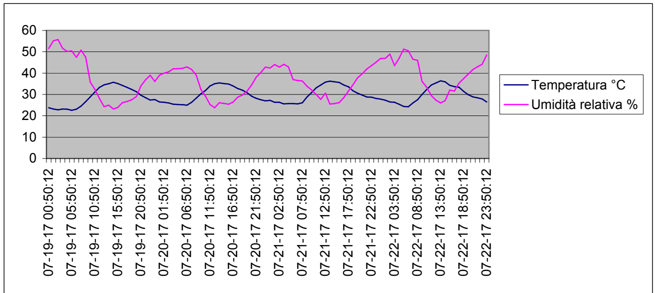
Grafico della temperature e dell'umidità relativa esterna dal 23-7-2017 al 31-7-2017
