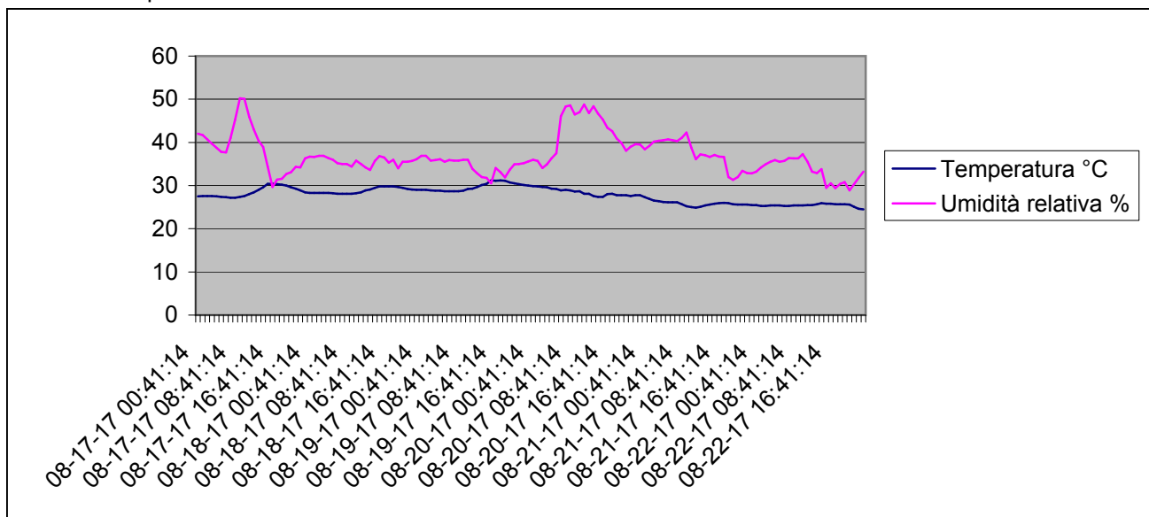
Grafico della temperature e dell'umidità relativa interna dal 17-8-2017 al 22-8-2017
