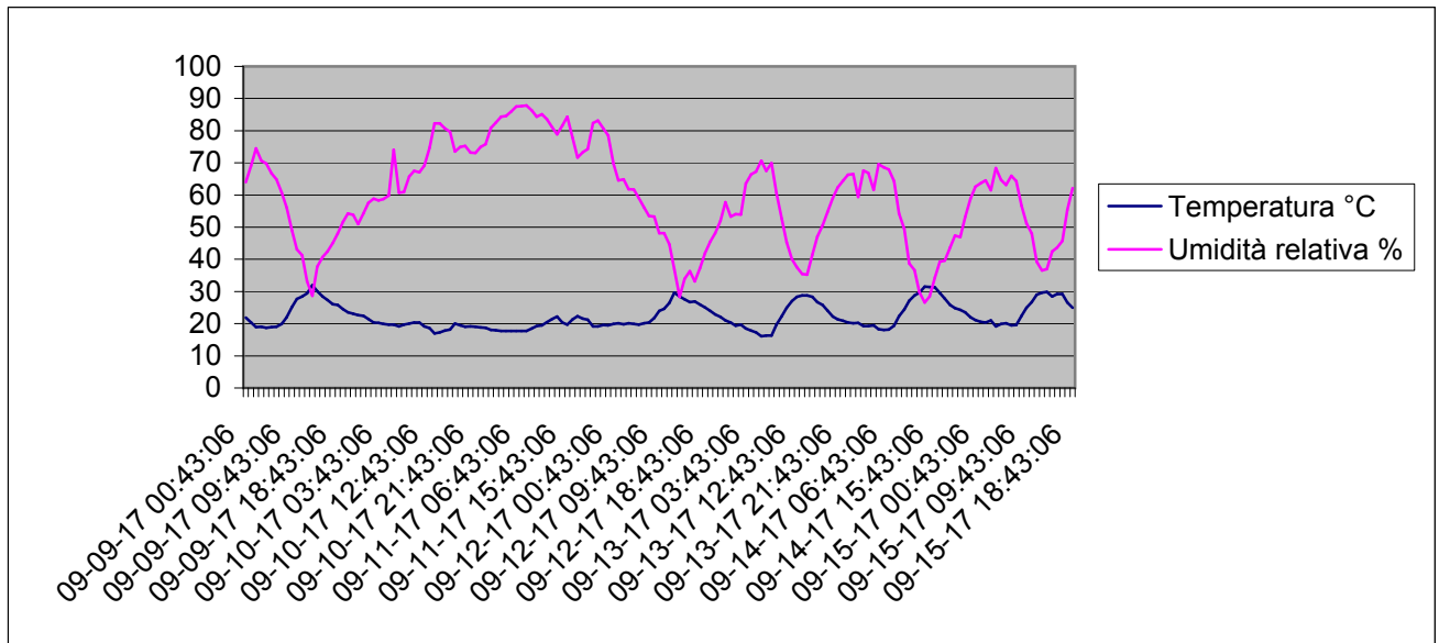
Grafico della temperature e dell'umidità relativa esterna dal 9-9-2017 al 15-9-2017
