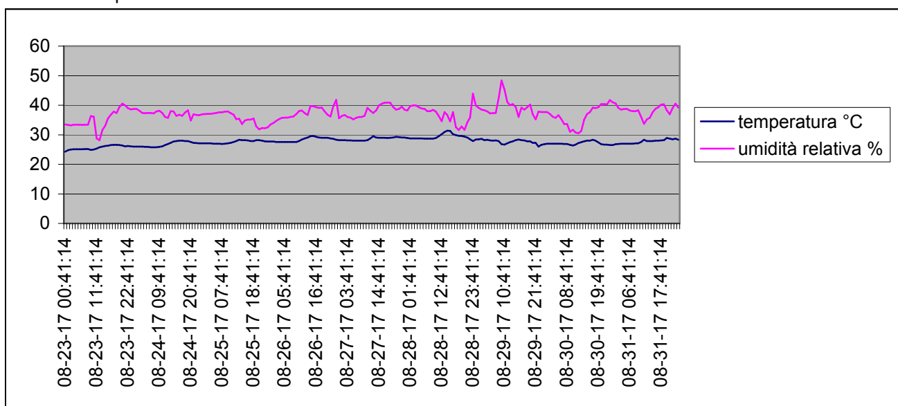
Grafico della temperature e dell'umidità relativa interna dal 23-8-2017 al 31-8-2017
