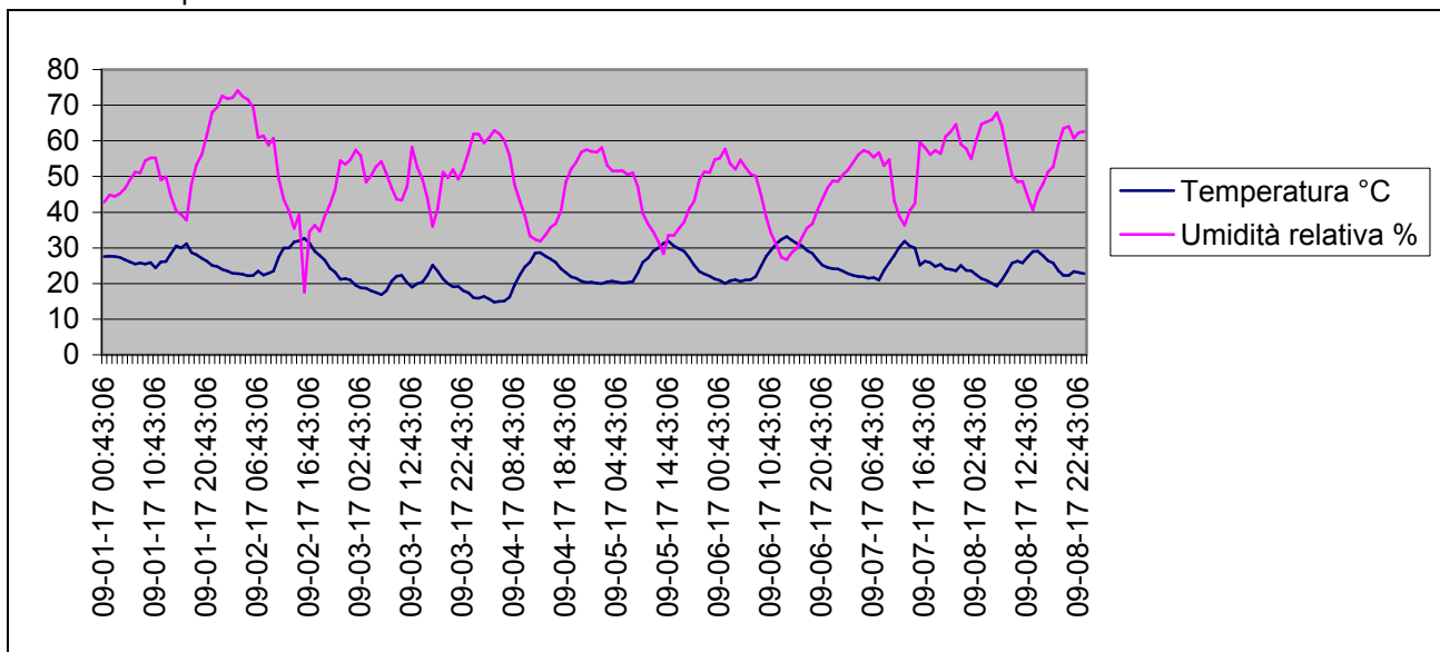
Grafico della temperature e dell'umidità relativa esterna dal 1-9-2017 al 8-9-2017
