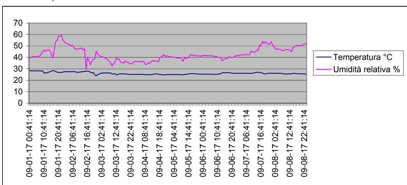
Grafico della temperature e dell'umidità relativa interna dal 1-9-2017 al 8-9-2017
