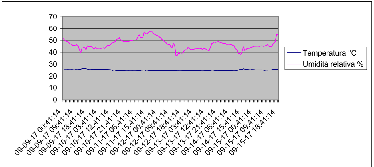
Grafico della temperature e dell'umidità relativa interna dal 9-9-2017 al 15-9-2017
