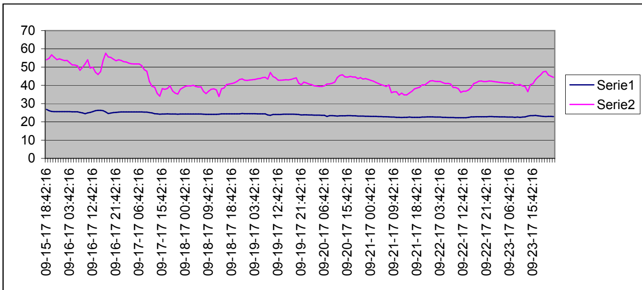
Grafico della temperature e dell'umidità relativa interna dal 15-09-2017 al 23-9-2017
