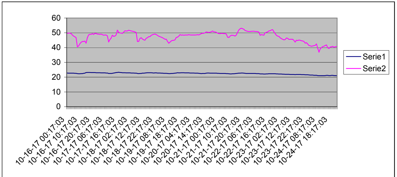
Grafico della temperature e dell'umidità relativa interna dal 16-10-2017 al 24-10-2017
