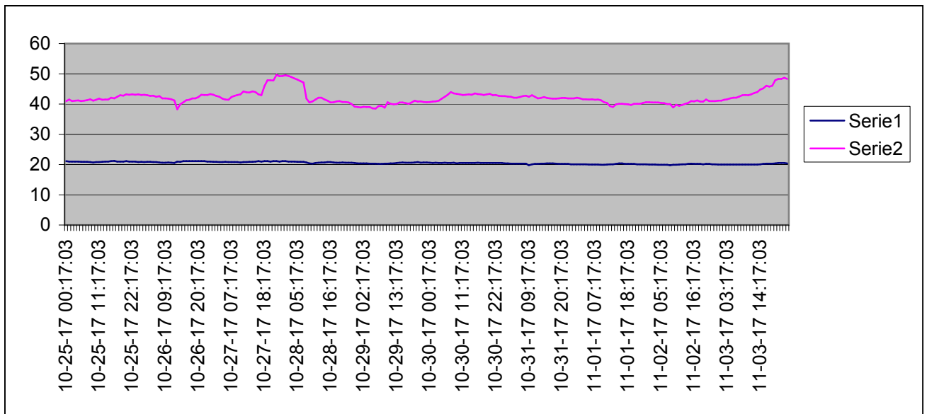
Grafico della temperature e dell'umidità relativa interna dal 25-10-2017 al 3-11-2017
