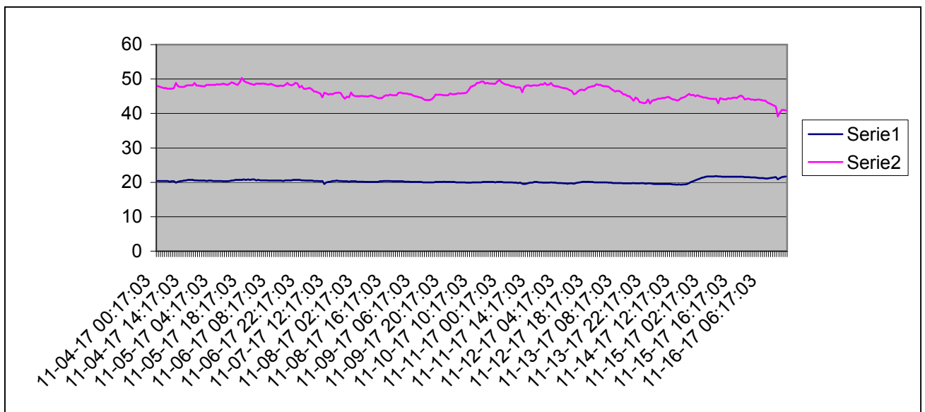
Grafico della temperature e dell'umidità relativa interna dal 4-11-2017 al 16-11-2017
