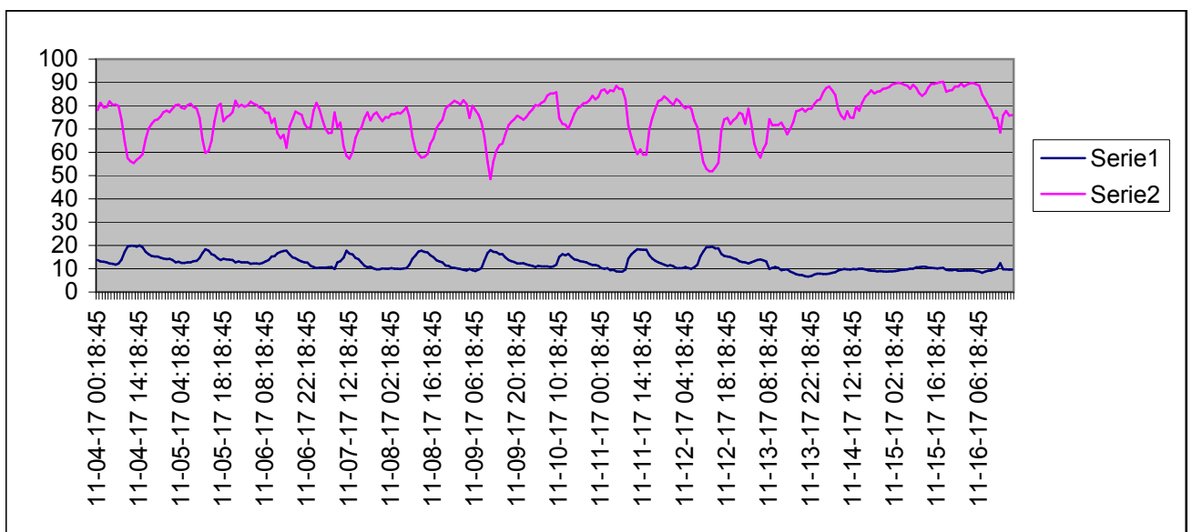
Grafico della temperature e dell'umidità relativa esterna dal 4-11-2017 al 16-11-2017
