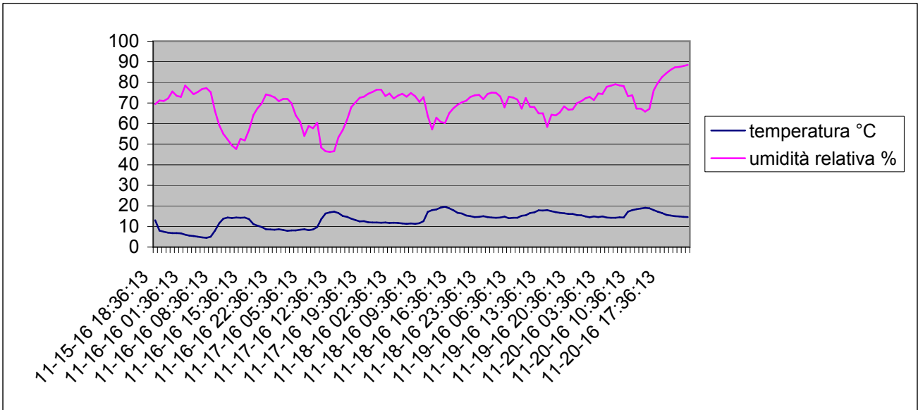
Grafico della temperature e dell'umidità relativa esterna dal 21-11-2016 al 27-11-2016
