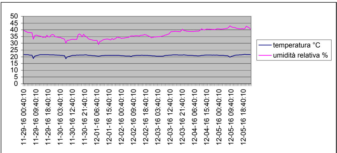
Grafico della temperature e dell'umidità relativa interna dal 29-11-2016 al 5-12-2016
