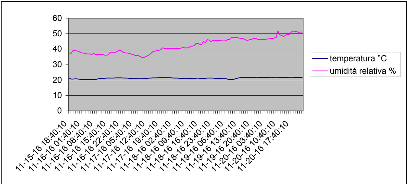
Grafico della temperature e dell'umidità relativa interna dal 15-11-2016 al 20-11-2016
