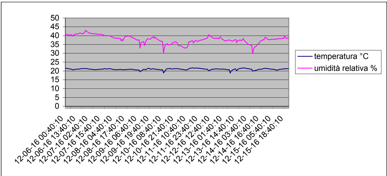
Grafico della temperature e dell'umidità relativa interna dal 6-12-2016 al 15-12-2016
