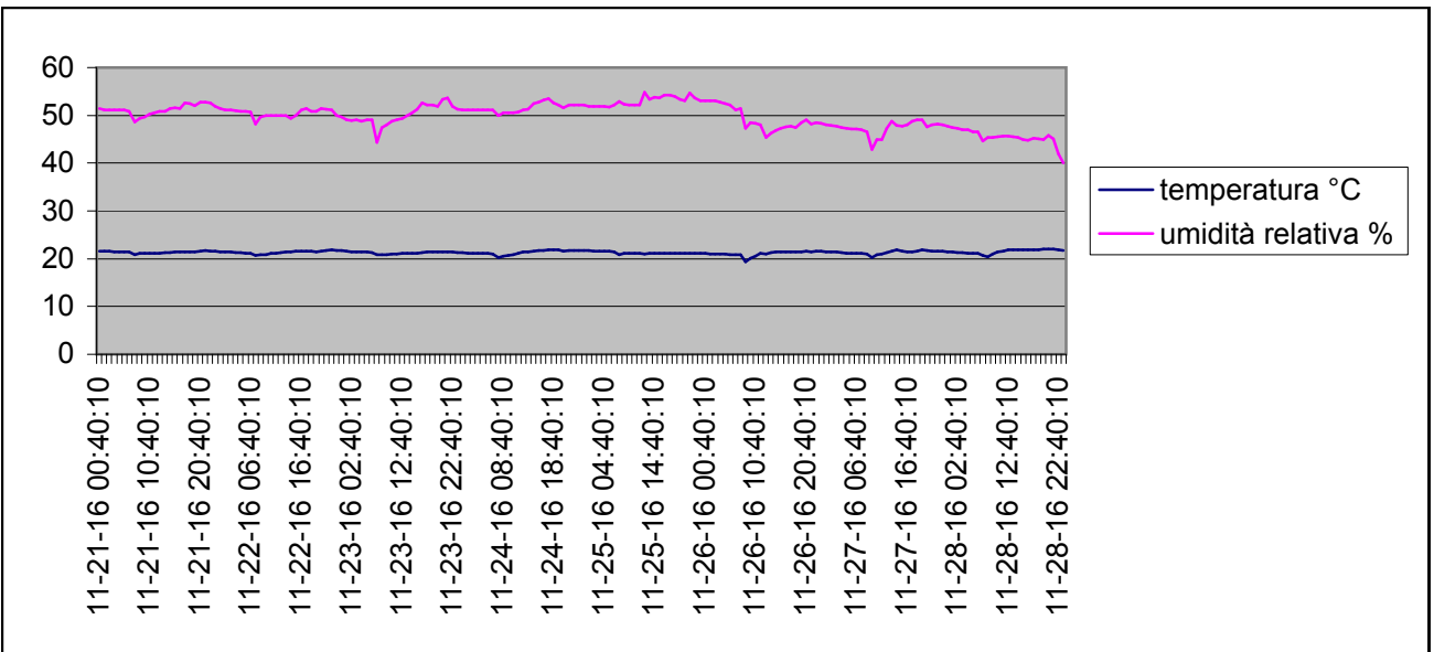
Grafico della temperature e dell'umidità relativa interna dal 21-11-2016 al 28-11-2016
