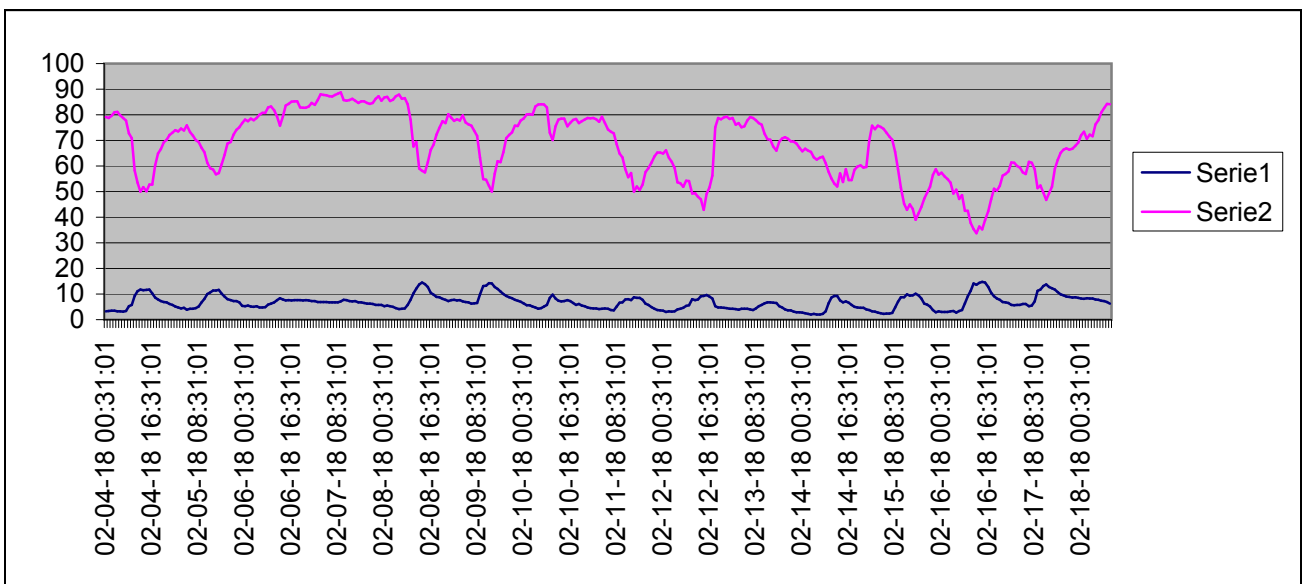
Grafico della temperature e dell'umidità relativa esterna dal 4-2 al 17-2-2018
