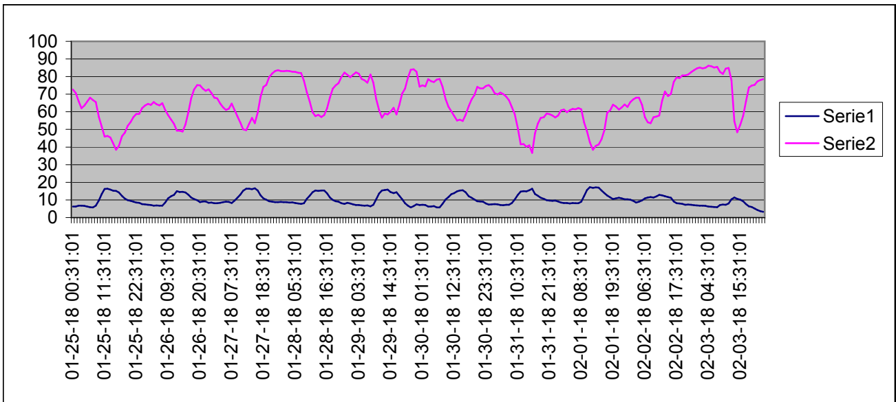
Grafico della temperature e dell'umidità relativa esterna dal 25-1 al 3-2-2018
