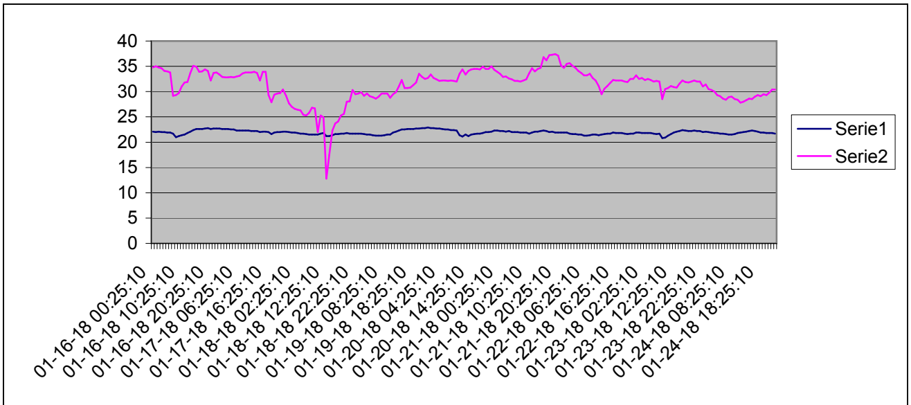
Grafico della temperature e dell'umidità relativa interna dal 25-1 al 3-2-2018
